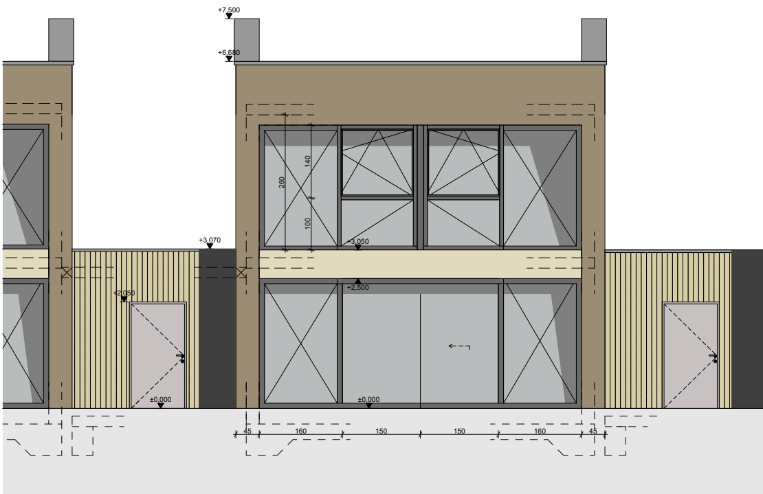
ANSICHT NORDOST M1:100
