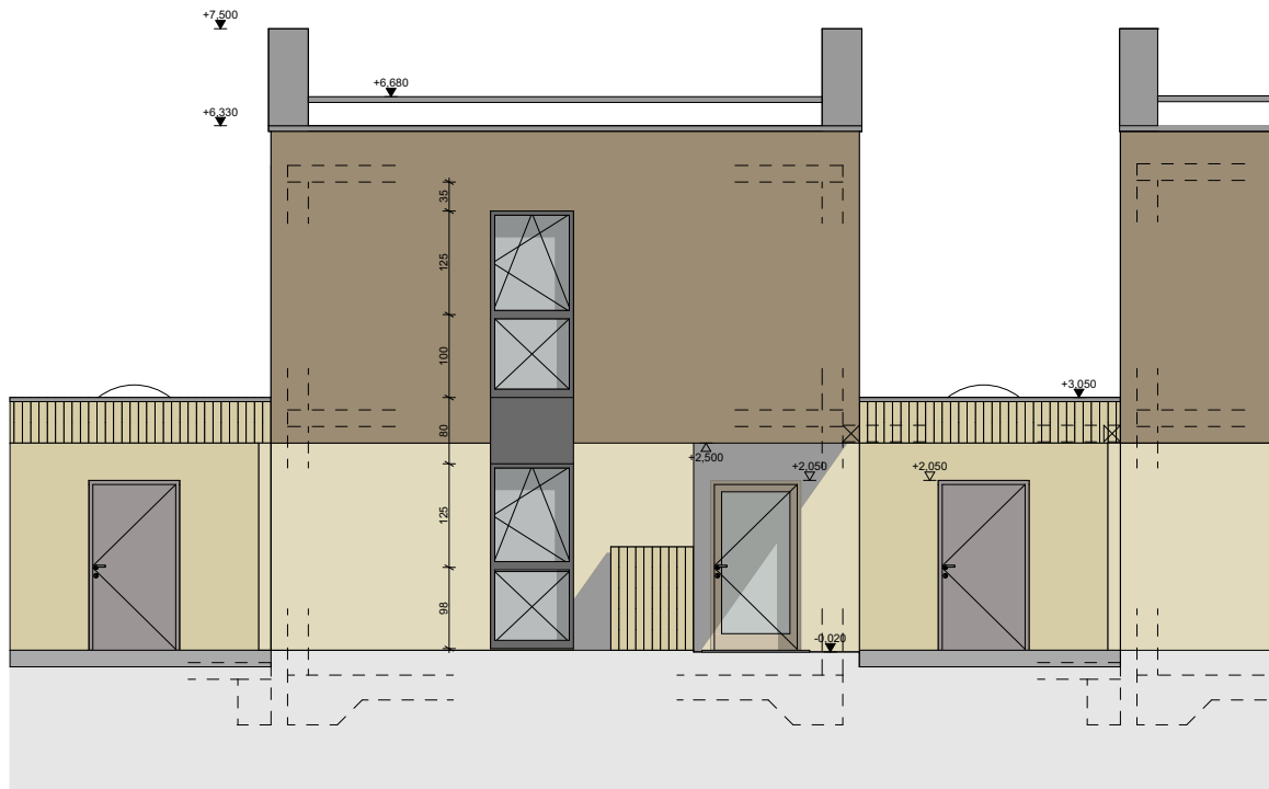
ANSICHT SÜDWEST M1:100
